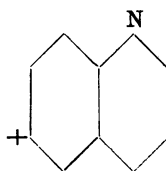
(Cleve.)
